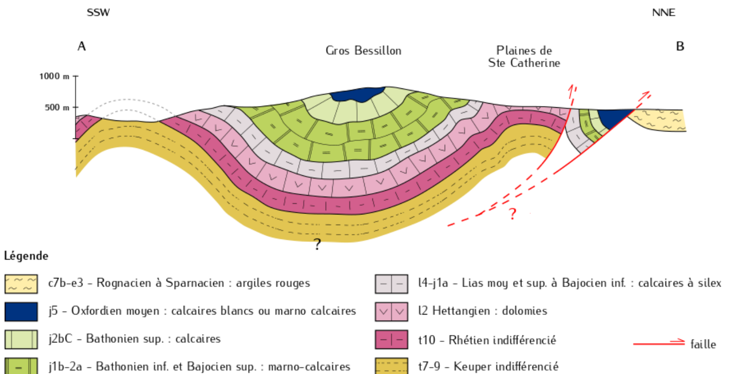
Coupe géologique à main levée de la carte de Brignoles initialement au 1/50 000
